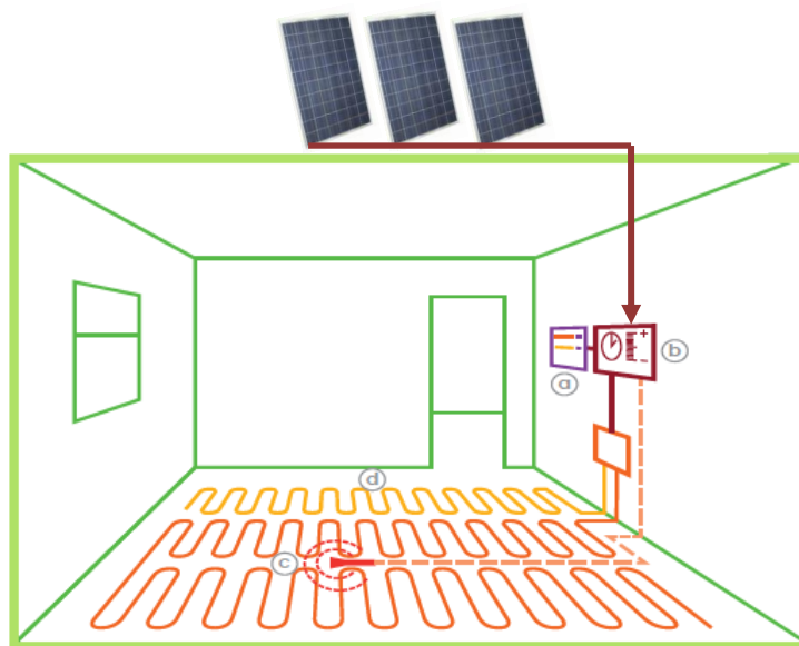
a) Centralina b) Crono-termostato c) Sonda di rilevazione d) Cavi scaldanti
